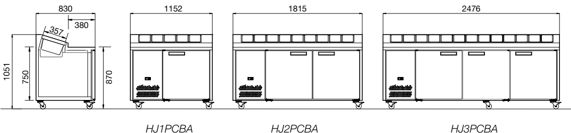
HJ1PCBA
